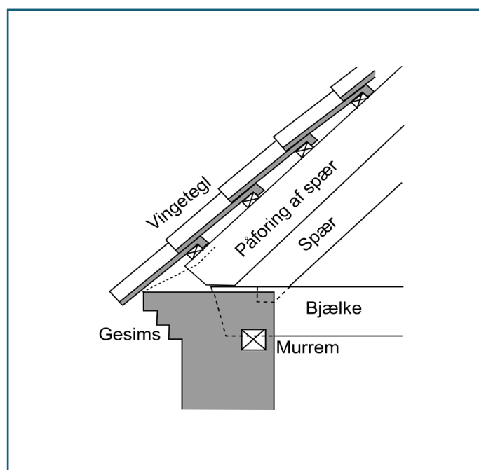
Renoveret tegltage, hvor skalken er erstattet af en påføring af spærhøjden afpasset, så forholdet mellem nederste tagsten og gesimsen forbliver uændret. Skematisk tværsnit i taggesims.
